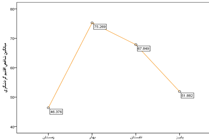
شکل ۳: میانگین شاخص فصلی TCI ایستگاه های مورد مطالعه در بازه زمانی ۲۰۱۶ تا ۱۹۸۶
