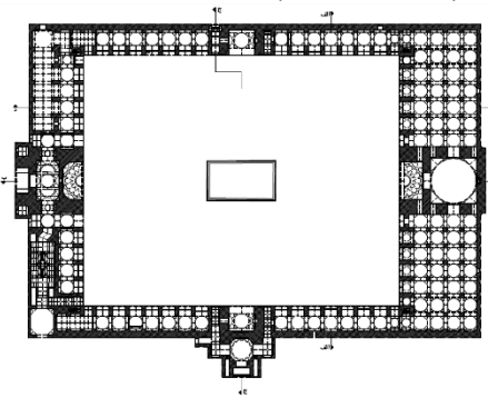
شکل ۴. پلان مسجد (آرشیو میراث فرهنگی استان قزوین)
